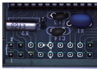
ハンダ無しとハンダ少の検出
